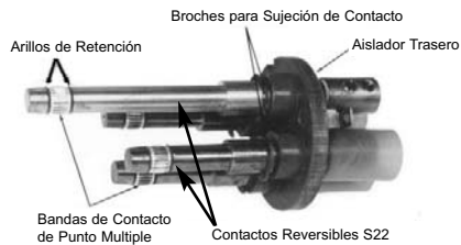
Figure 10. Sufijo S22 - Contactos invertidos
