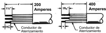
Figure 5. Aislamiento del cable
