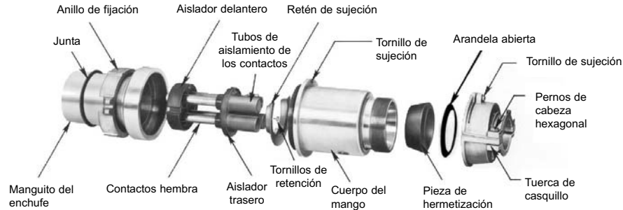
Figure 1 - Descripción detallada del enchufe AP (Tipo 2 mostrado)
