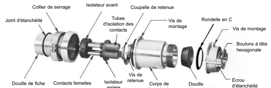
Figure 1 - Description détaillée d'une fiche AP (fiche de style 2 représentée)
