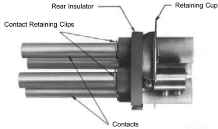
Figure 8. Position des clips de retenue
