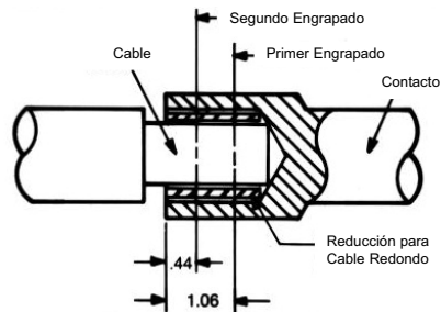
Figure 7. Conexión por engarzado a presión
