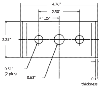
DSXF1 DSXF2 YOKE
