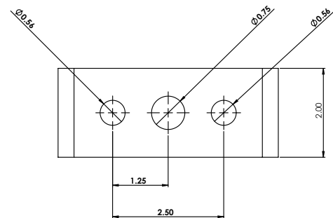
DSXF3 YOKE
