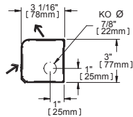
CÔTÉ | SIDE
