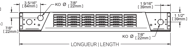
DESSUS | TOP
