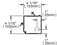
CÔTÉ | SIDE
