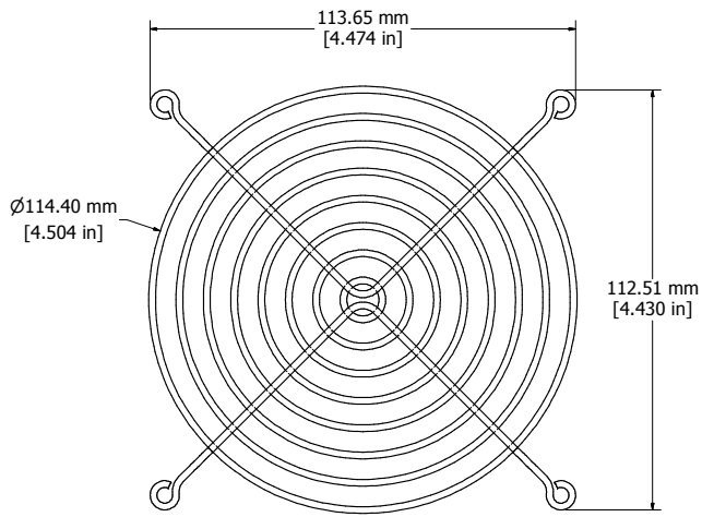
FAN GUARD TOP VIEW (2X)
