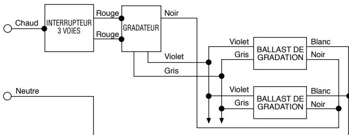
Figure 2 – câblage 3 voies
