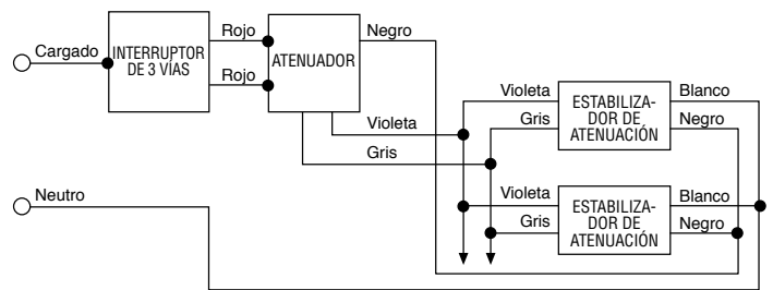
Figura 2 – Cableado de 3 vías
