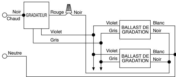
Figure 2 – câblage 3 voies
