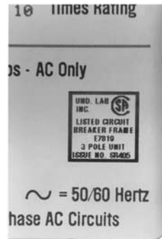
UL Label
