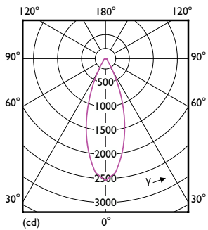
LEDspots N DIM 13W PAR38 E26 930 40D-LDD
