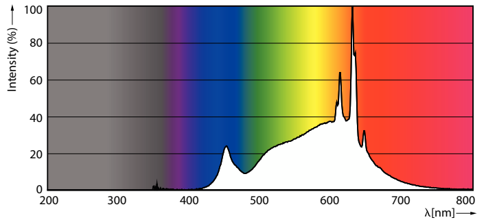
LEDspots N DIM 13W PAR38 E26 930 40D-POC
