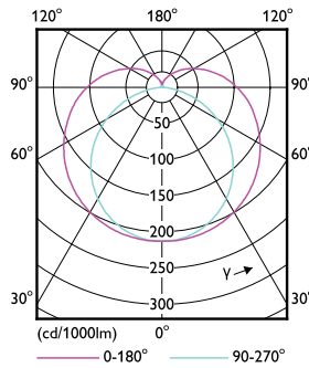
LEDtube 14W G13 2000lm
