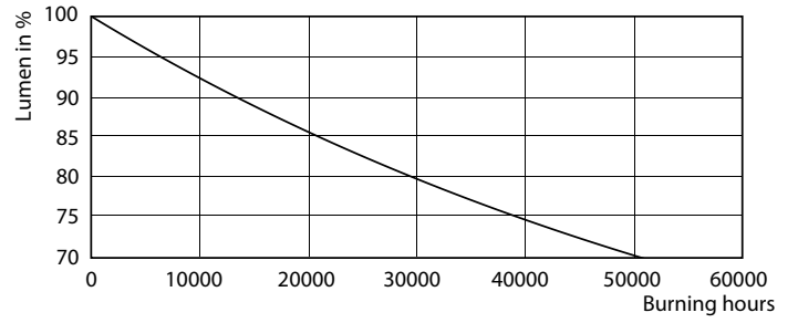
LEDspot 50W GU10 830 35D
