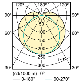
LEDtube 900 mm 10.5 W /830
