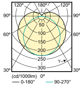
LEDtube 600 mm 8.5 W /850
