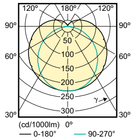
LEDtube 600 mm 8.5 W /840
