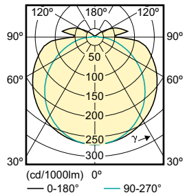
LEDtube 600mm 16.5 W
