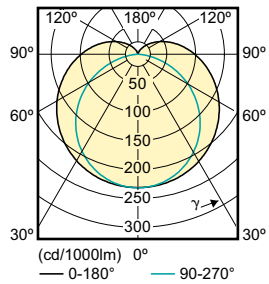
LEDtube 900 mm 10.5 W /835
