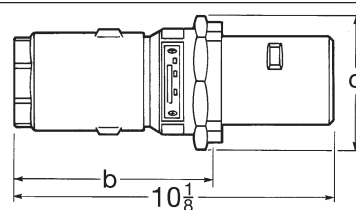
APJ Plug
