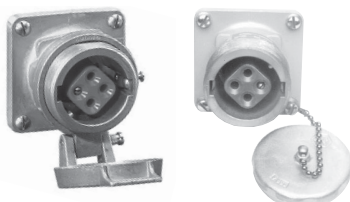
Receptacle
