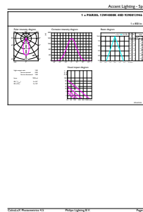
LEDspot 12-75W E26 PAR30L 840 850lm 40D
