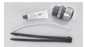
ELVB-SRA(x)-34-ST
